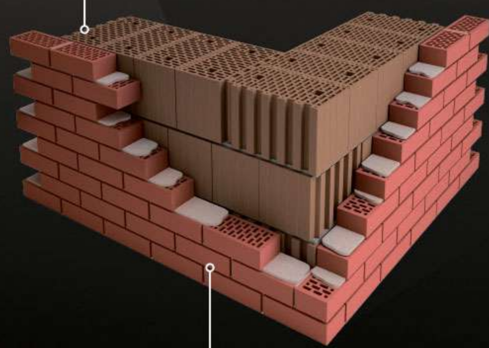
Облицовочный кирпич
