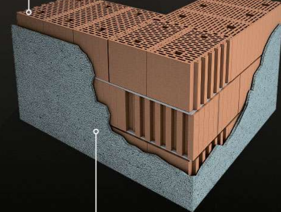
Фасадная штукатурка
